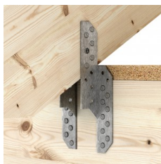
Fijación de pie de cabrio con forjado
