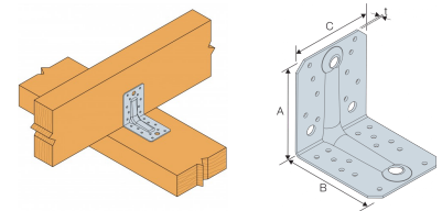
Fixation bois/bois
