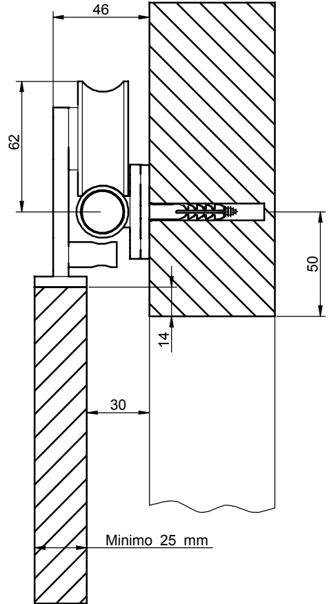
FIJACION TRASERA PARED / Back fixing wall / Fixation l'arriere sur mur
