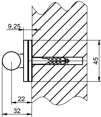
FIJACION TRASERA PARED / Back fixing wall / Fixation l'arriere sur mur
