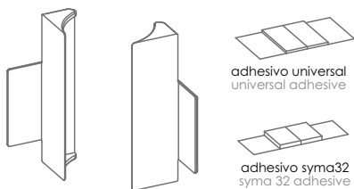
personalizable con lámina plana (ancho 31mm; grueso < 3 mm) customizable with flat sheet (width 31mm; thickness < 3mm)
